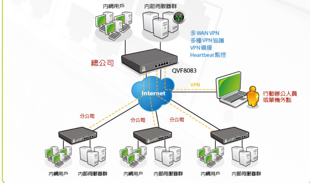
QVF8083應用方案示意圖
