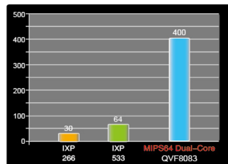
64Byte封包轉發效能
